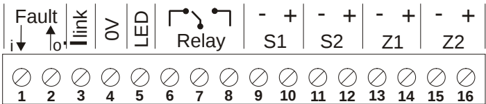
Figur 3: Inngang/utgang terminaler
