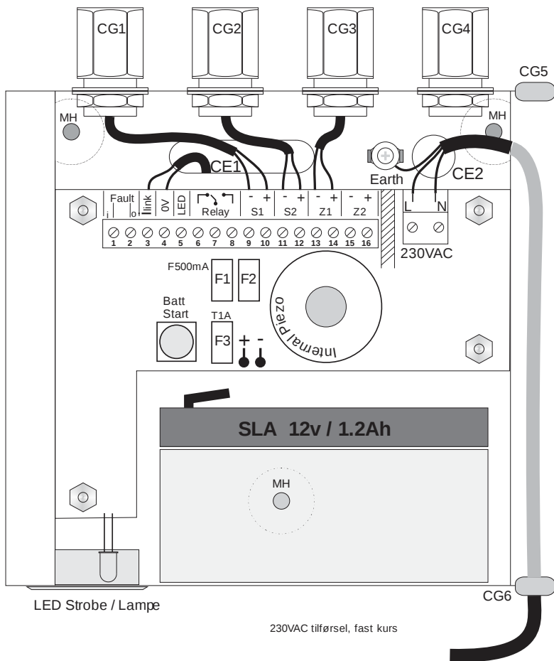
Figur 2: Kretskort
