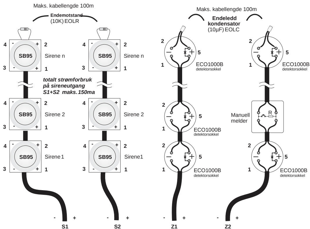
Figur 1: Detektor og sirenekobling
