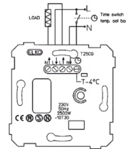
Koblingsskjema
