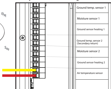
Detaljoversikt tilkobling
