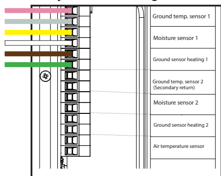
Detaljoversikt tilkobling
