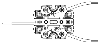
Koblingskjema
