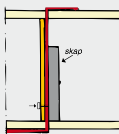
Fig. 3 Vertikal rørføring
