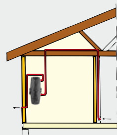
Fig. 4 Føring i loft
