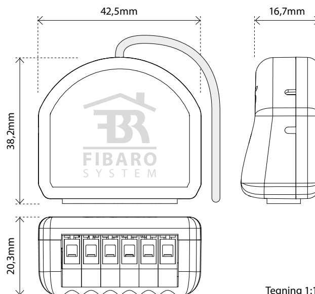
Tegning 1:1
