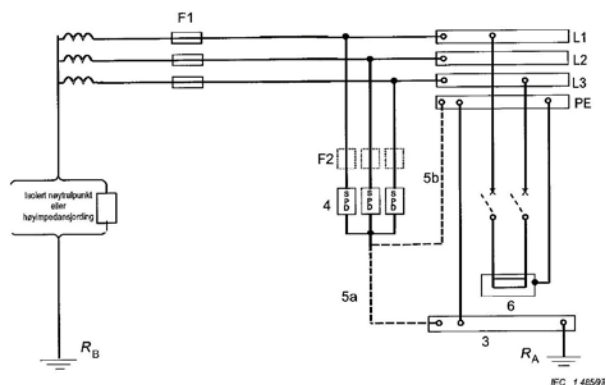
Overspenningsvern i et IT-system
