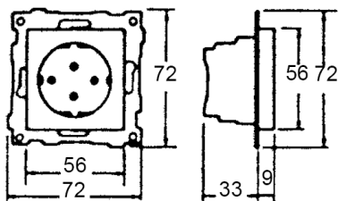
Målskisse
