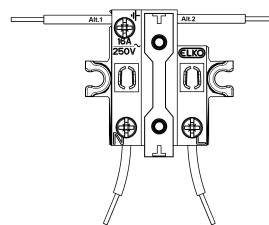
Koblingsskjema
