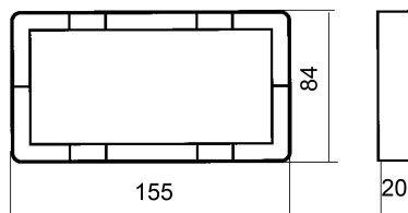
Målskisse
