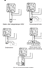
Koblings skjema
