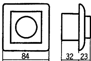
Målskisse
