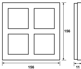
Målskisse
