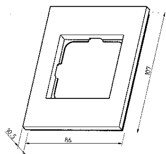
Målskisse
