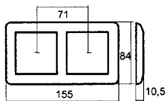
Målskisse
