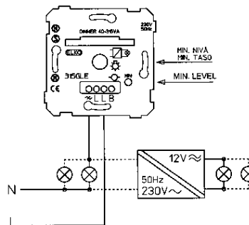
Koblingsskjema
