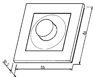
Målskisse
