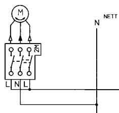
Koblingsskjema
