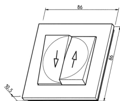
Målskisse
