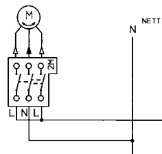
Koblingskjema
