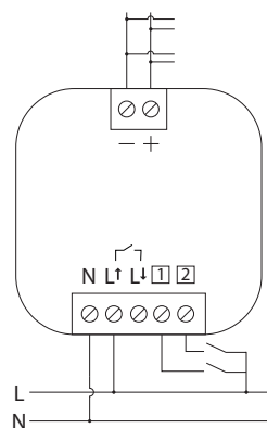
Kobling for 0-10 V buss (uten avbrudd av forsyning til last)
