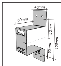
Brakett
