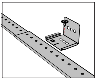
Monter Skive (EL NR.13 428 17) på teleskopet med Ø 4,2mm skrue.
