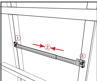
1. Skru fast. 2. Juster så hullene er ovenfor hverandre. 3. Skru fast andre siden.
