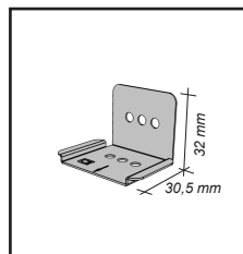
Skive
