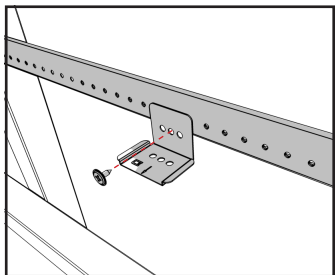
Monter skive EL.NR 13 428 17 med Ø 4,2mm skrue. Pass på eventuell plast i bakkant.
