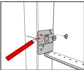
Indikert pil markerer hvor boksens senter vil være. Monteres i kant på stender og skrues fast i begge sider.
