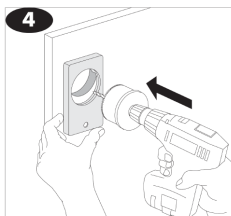
Malen styrer hullfresen ved utfresing av halvmånen
