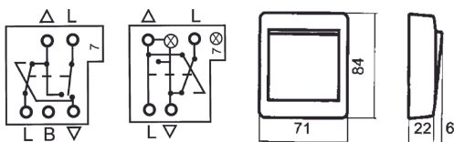
Kryssvender (7)
