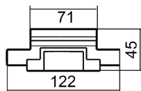
Veggbox hvit S45
