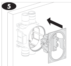
Lav stikkontakt tilkobles. Dersom du skal benytte multiboks 1,5 skal denne monteres før tilkobling.
