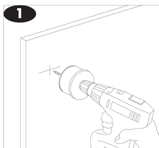
Veggplate merkes og borres med 73mm hullfres
