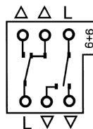
Kobling 6+6 Dobbel veksel- vender
