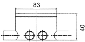
Takboks 40mm høyde
