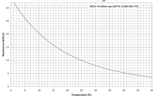
Motstandsverdier for NTC gulvføler
