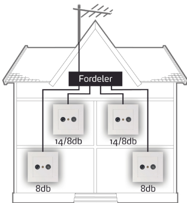
Flere abonnenter (stjernenett) med felles antenne eller kabel-TV.
