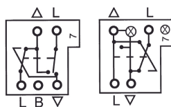
Kryssvender (7)
