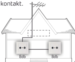
Eksempel på serienett
