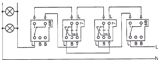
Kryssvender (7)
