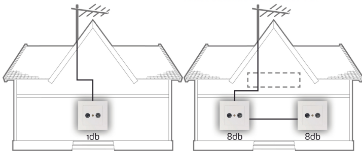
Pr. abonnent (enkeltnett) for en husstand eller pr. leilighet i blokk.
