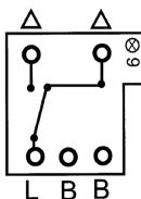
Kobling 6 Vekselvender
