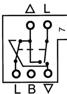
Kobling 7 Kryssvender
