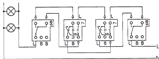
Kryssvender (7)
