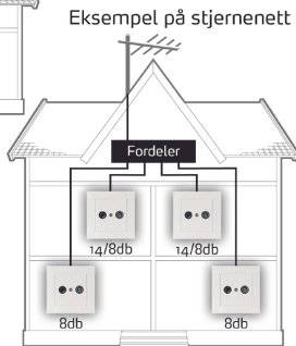
Eksempel på stjerne-nett
