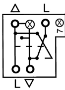
Kobling 7 Lys Kryssvender med lys
