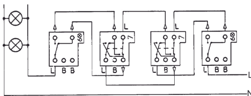
Kryssvender (7)
