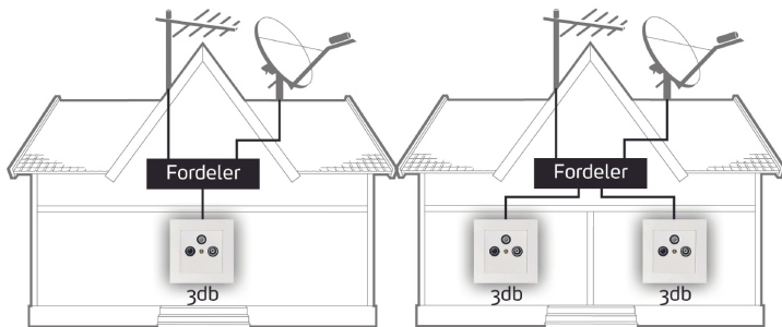
Antenne/satelittkontakter, en eller to abonnemeter.
