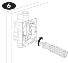
Lav stikkontakt monteres sentrisk i veggboksen
