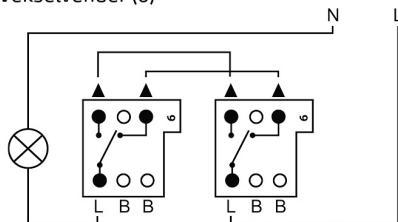
Vekselvender (6)
