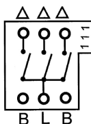
Kobl 1+1+1 3x1 Polet
