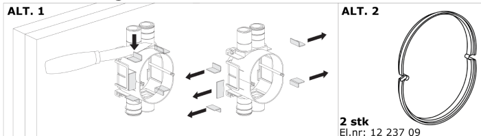
Lav stikkontakt tilkobles. Dersom du skal benytte multiboks 1,5 skal denne monteres før tilkobling.
